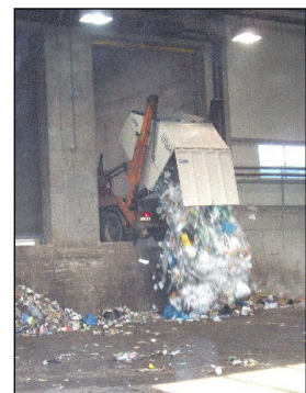
Abkippkante
