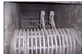
Hammermühle Innenansicht
