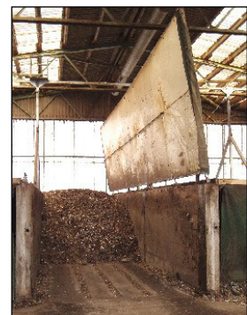
Intensivrotteboxen
