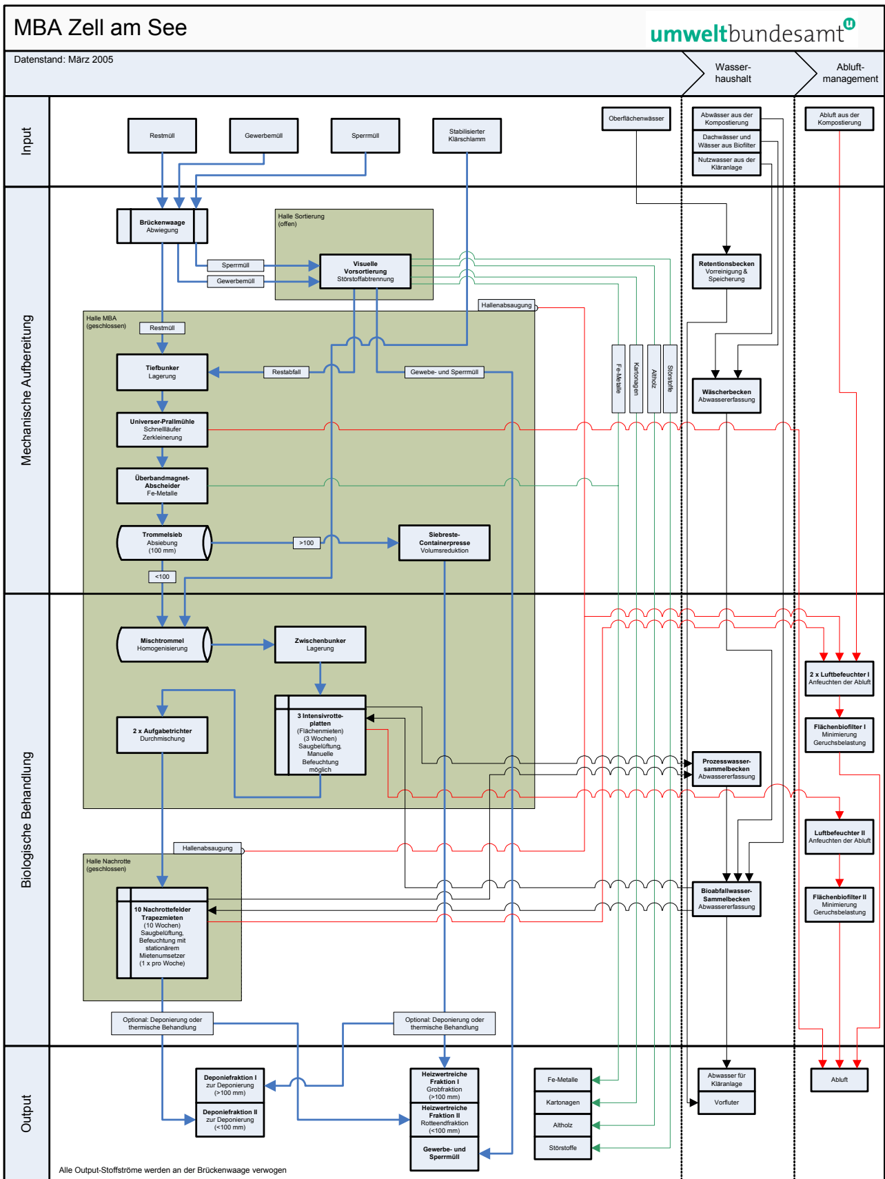
Abbildung 17: Ablaufschema der MBA Zell am See.
