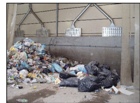
Tiefbunker
