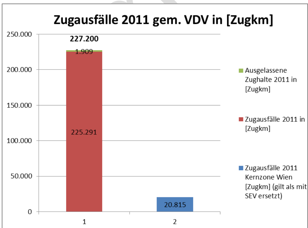
Abbildung 6: ausgefallene Leistungen bei ÖBB-PV AG
