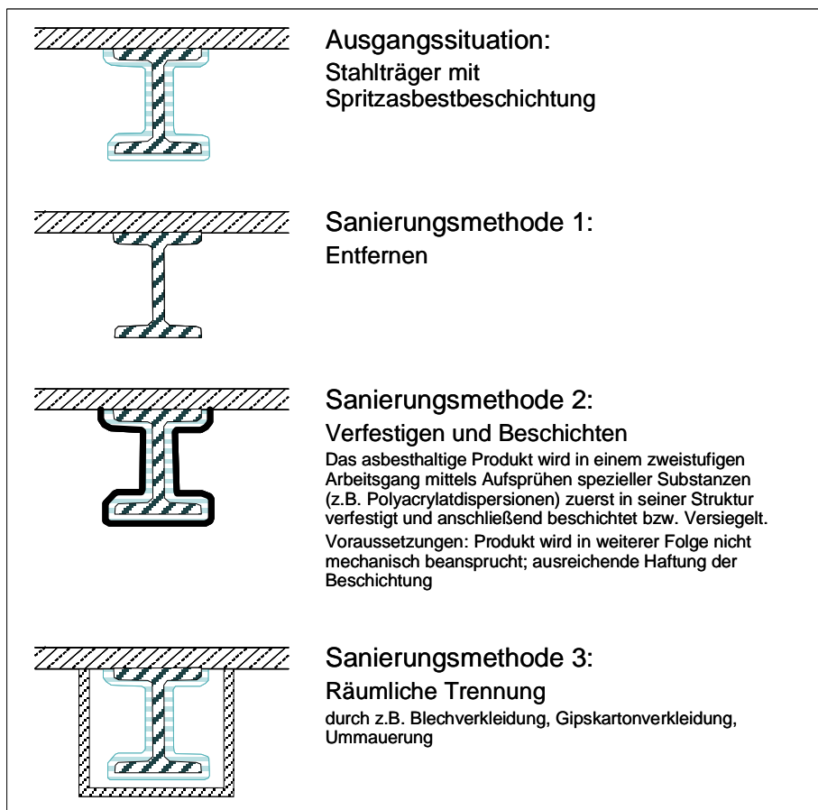
Abbildung 4: Methoden der Asbestsanierung (DWORAK 2002)
