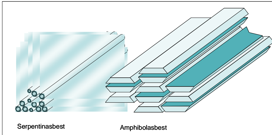
Abbildung 3: Faserstruktur der Asbeste (nach DWORAK 2002)
