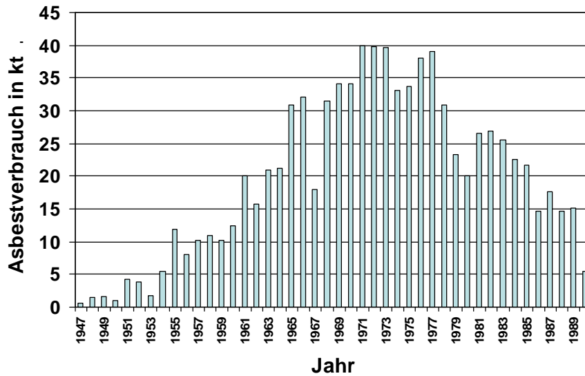
Abbildung 1: Asbestverbrauch in Österreich (DWORAK 2002)
