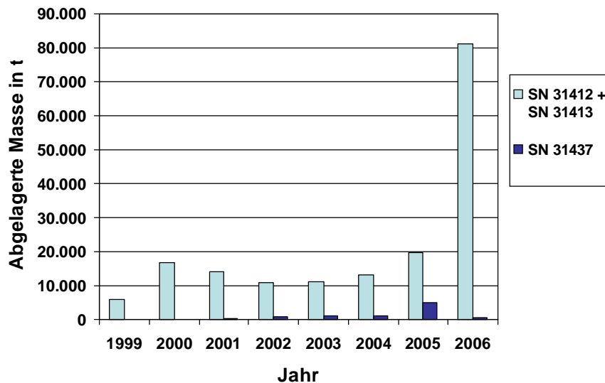
Abbildung 2: Auf Deponien abgelagerte Asbestabfälle in Österreich (Auswertung aus der Anlagen- und Stoffdatenbank des Umweltbundesamtes, Datenstand 6.11.2007) (SN 31412 Asbestzement, SN 31413 Asbestzementstäube, SN 31437 Asbestabfälle, Asbeststäube)
