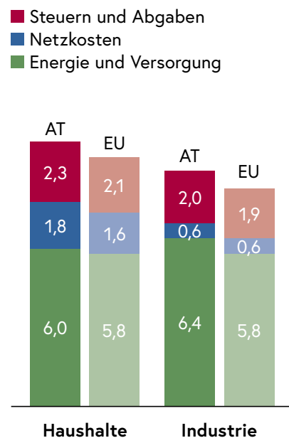
Abb. 56: Gaspreise für Industrie und Haushalte 2022 nach Komponenten in Cent/kWh
