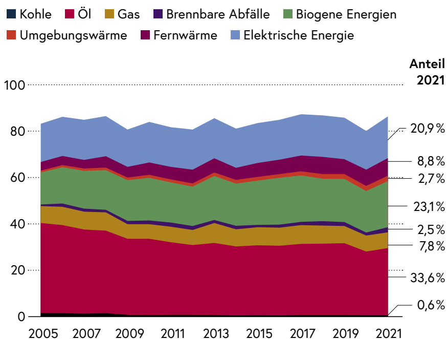
Abb. 65: Energetischer Endverbrauch (EEV) in Kärnten nach Energieträgern in Petajoule 2005–2021
