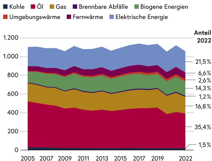
Abb. 16: Energetischer Endverbrauch nach Energieträgern in Petajoule 2005–2022
