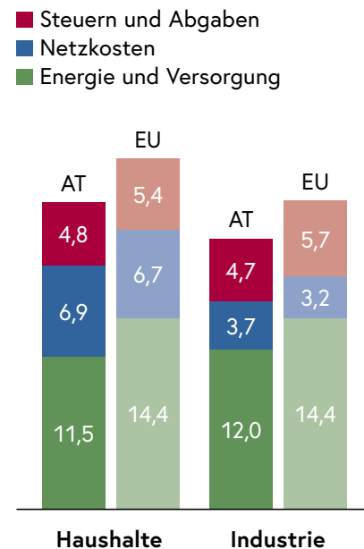
Abb. 54: Strompreise für Industrie und Haushalte 2022 nach Komponenten in Cent/kWh
