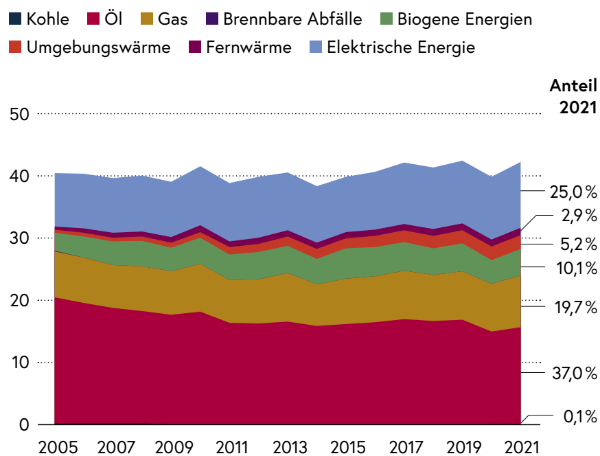
Abb. 77: Energetischer Endverbrauch (EEV) in Vorarlberg nach Energieträgern in Petajoule 2005–2021
