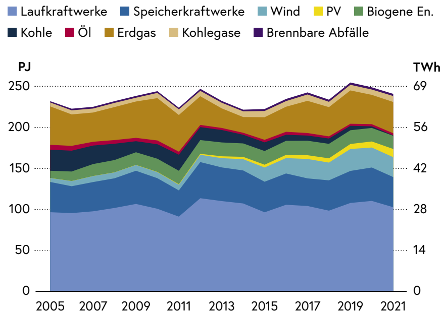
Abb. 14: Bruttostromerzeugung in Österreich in PJ (linke Skala) und TWh (rechte Skala) 2005–2021*
