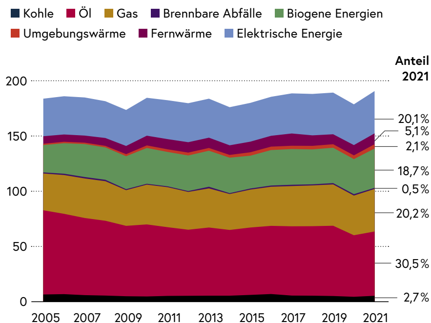
Abb. 73: Energetischer Endverbrauch (EEV) in der Steiermark nach Energieträgern in Petajoule 2005–2021
