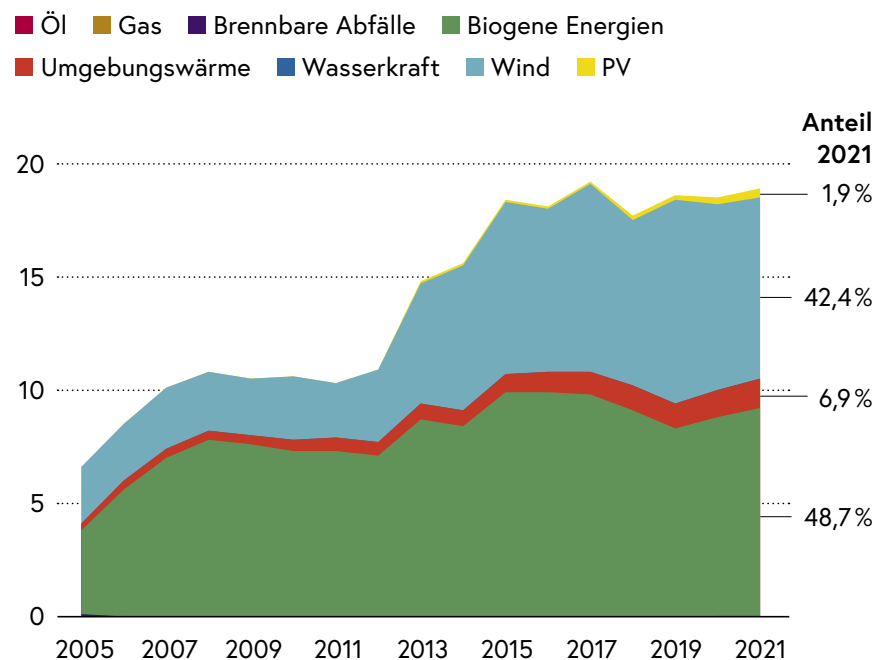
Abb. 62: Primärenergieerzeugung (PE) im Burgenland nach Energieträgern in Petajoule 2005–2021
