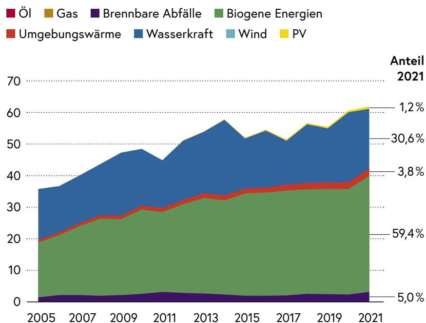
Abb. 64: Primärenergieerzeugung (PE) in Kärnten nach Energieträgern in Petajoule 2005–2021
