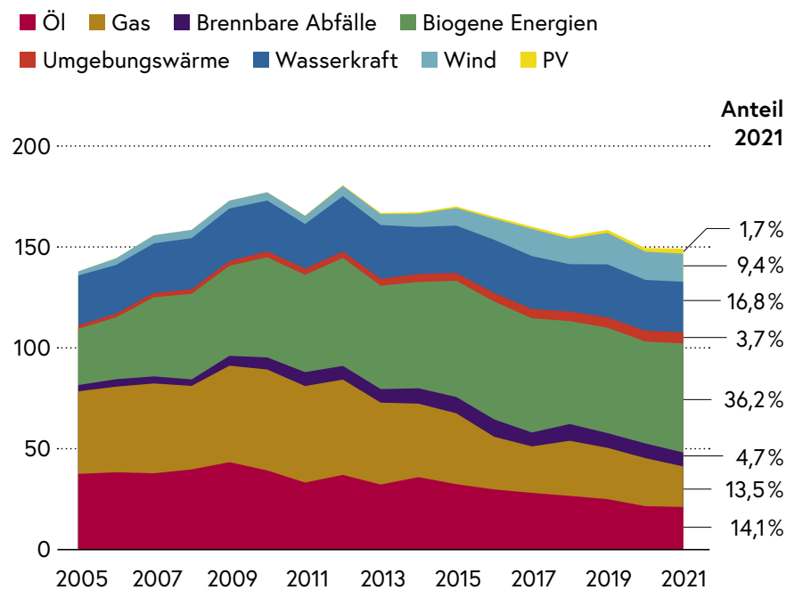
Abb. 66: Primärenergieerzeugung (PE) in Niederösterreich nach Energieträgern in Petajoule 2005–2021
