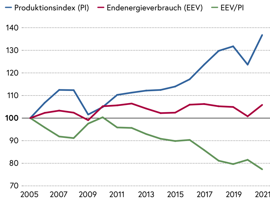
Abb. 38: Energieintensität der Industrie
