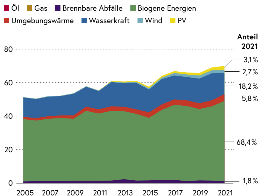
Abb. 72: Primärenergieerzeugung (PE) in der Steiermark nach Energieträgern in Petajoule 2005–2021
