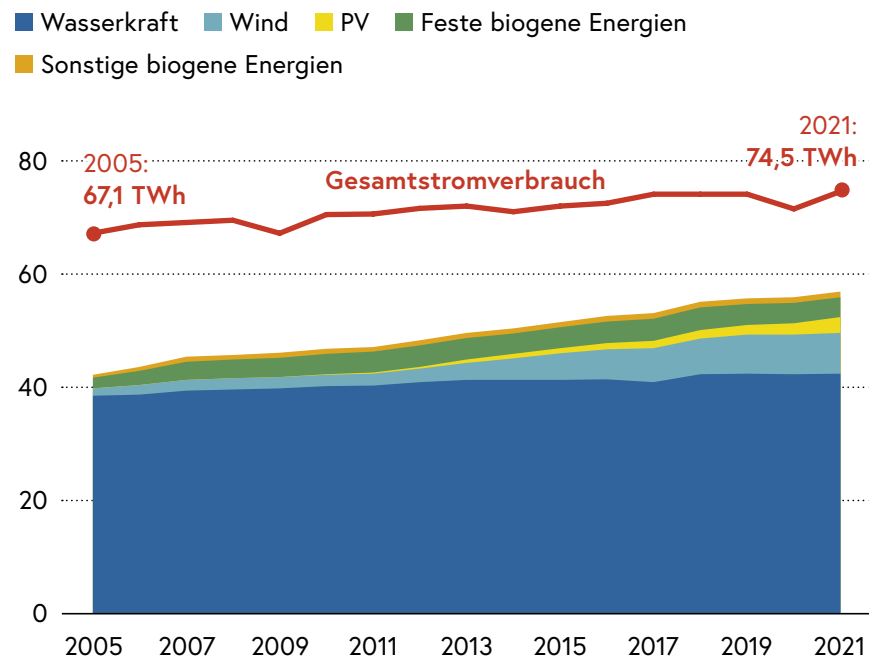
Abb. 26: Erneuerbarer Strom 2005–2021 in Relation zum Gesamtstromverbrauch in TWh
