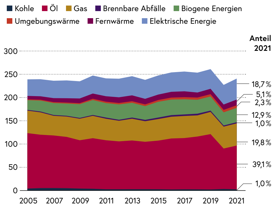
Abb. 67: Energetischer Endverbrauch (EEV) in Niederösterreich nach Energieträgern in Petajoule 2005–2021
