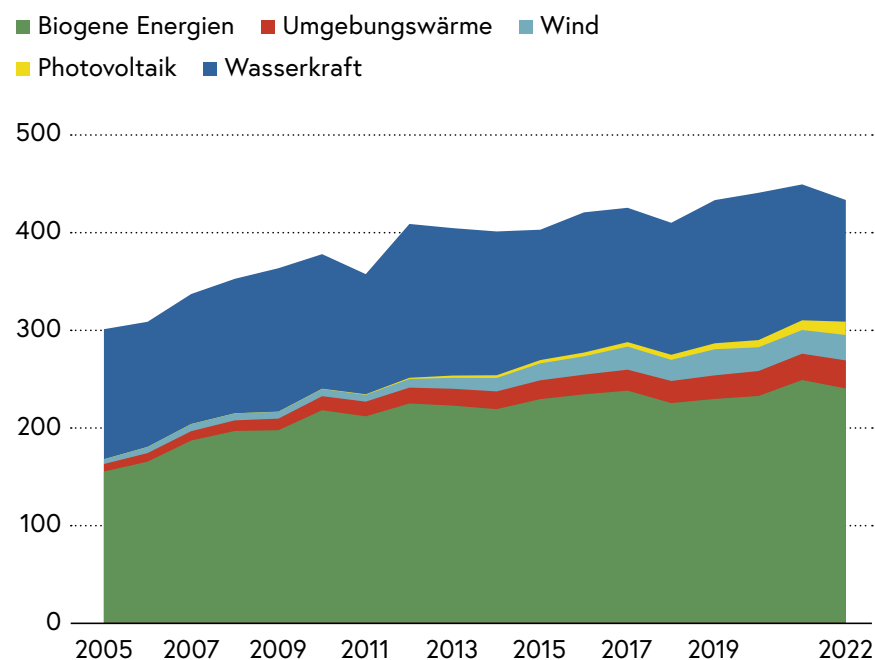
Abb. 18: Erzeugungsstruktur der erneuerbaren Energien in Österreich 2005–2022 in Petajoule
