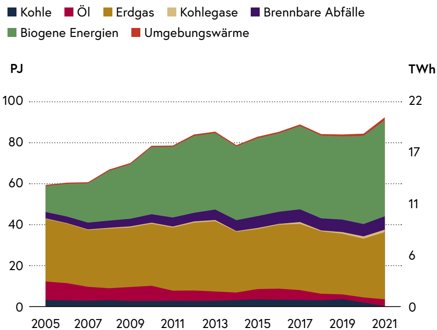
Abb. 15: Fernwärmeerzeugung nach Energieträgern in PJ (linke Skala) und TWh (rechte Skala) 2005–2021*
